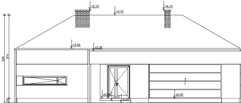
ELEWACJA FRONTOWA
