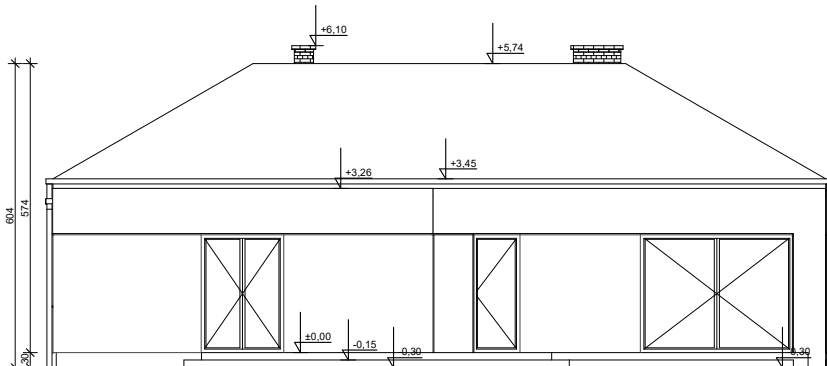
ELEWACJA OGRODOWA
