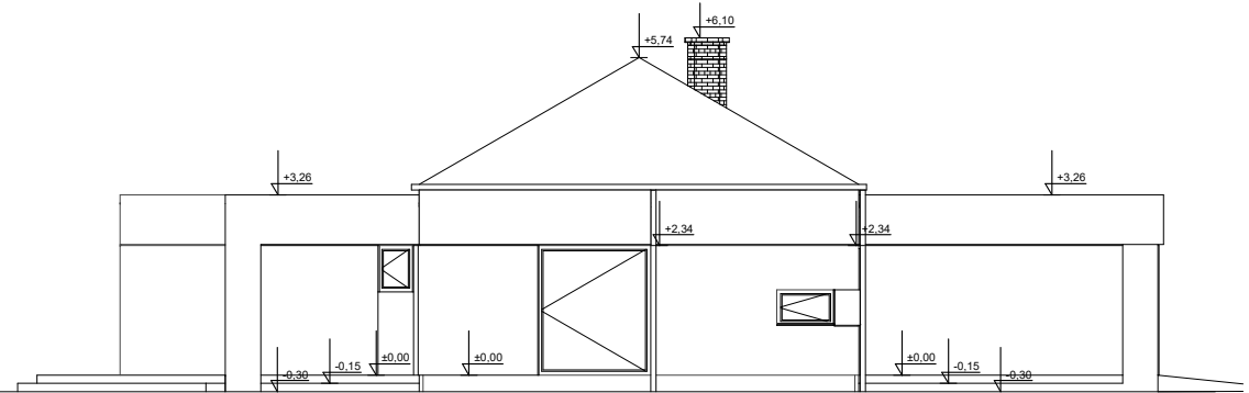
ELEWACJA BOK 1
