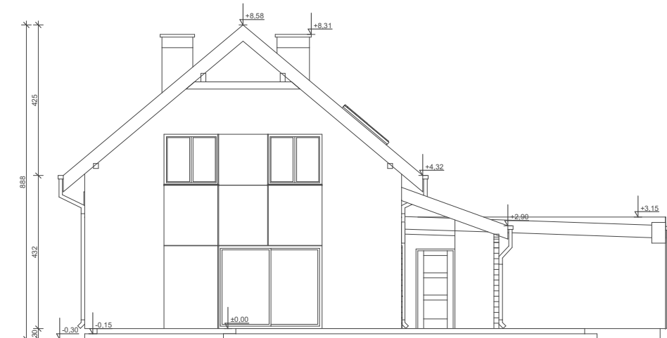
ELEWACJA OGRODOWA
