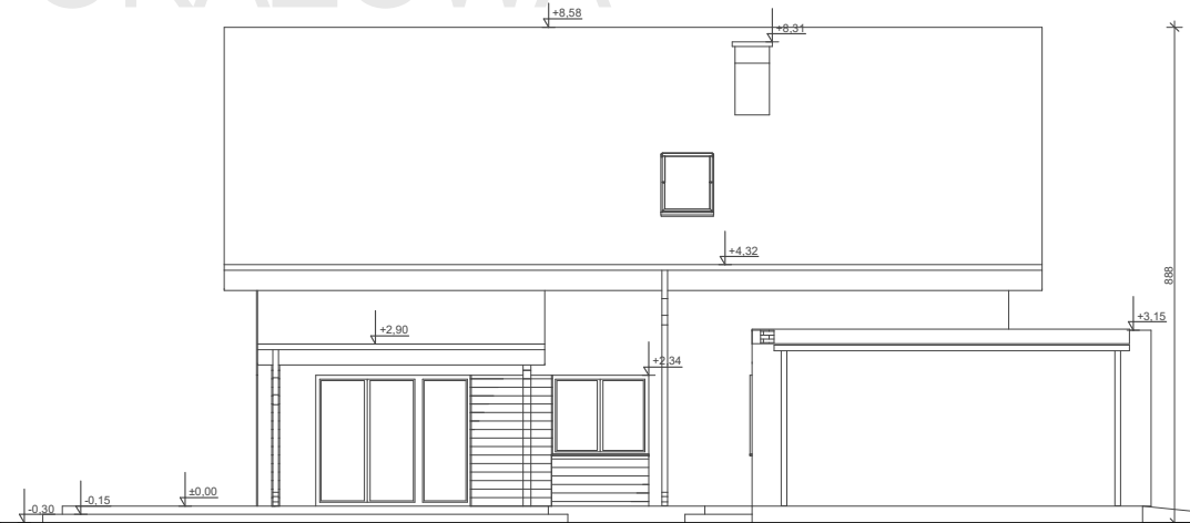
ELEWACJA BOK 1
