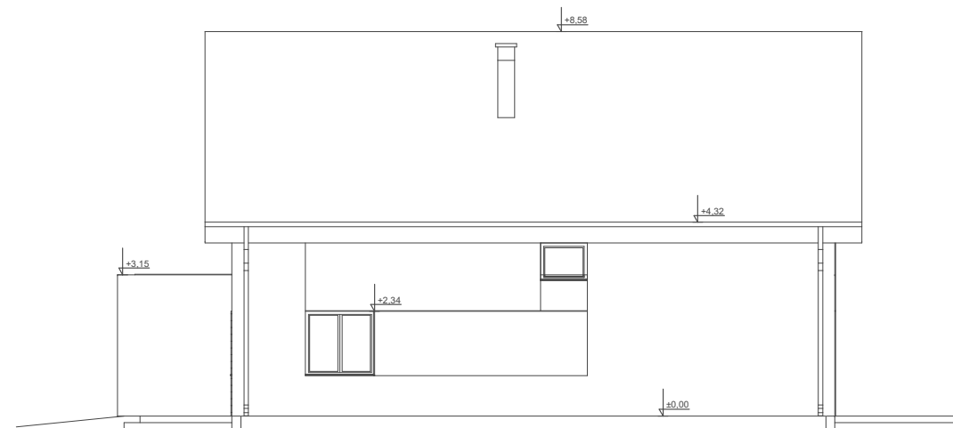
ELEWACJA BOK 2
