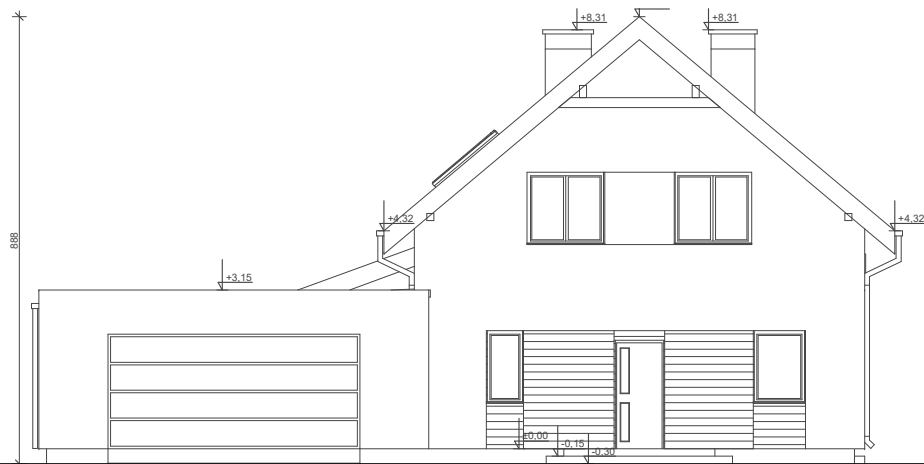
ELEWACJA FRONTOWA
