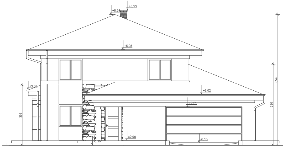
ELEWACJA FRONTOWA
