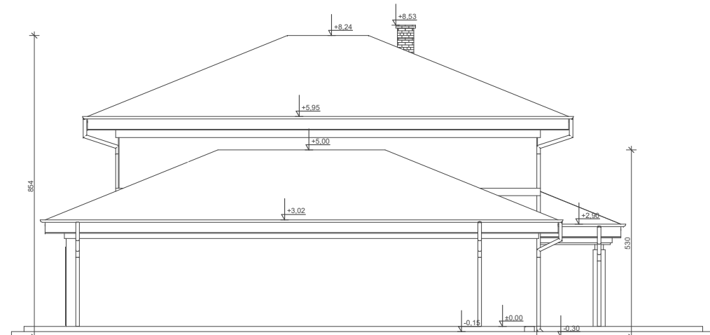
ELEWACJA BOK 2
