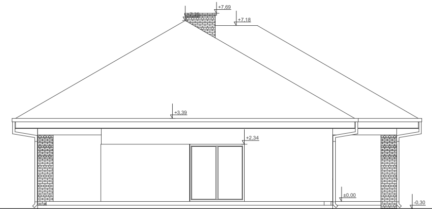
ELEWACJA BOK 1
