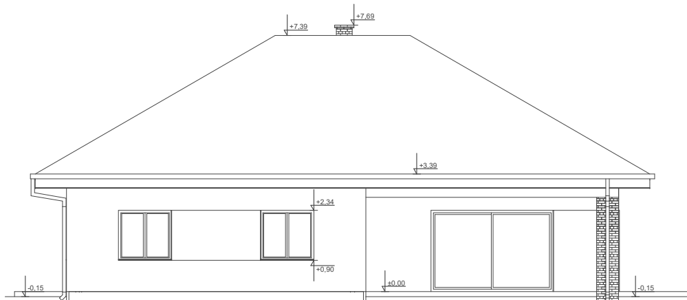
ELEWACJA OGRODOWA
