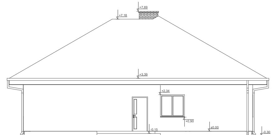
ELEWACJA BOK 2
