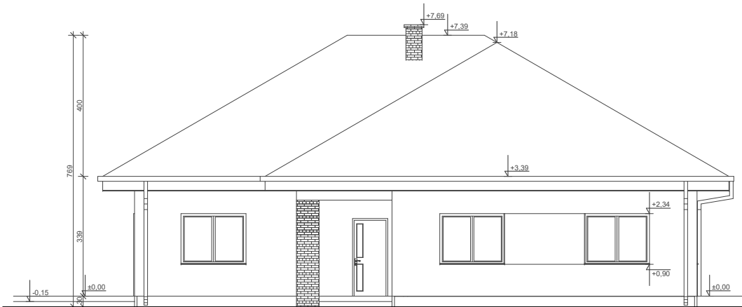
ELEWACJA FRONTOWA
