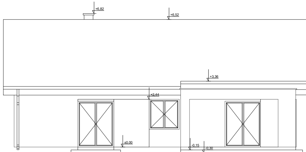
ELEWACJA OGRODOWA
