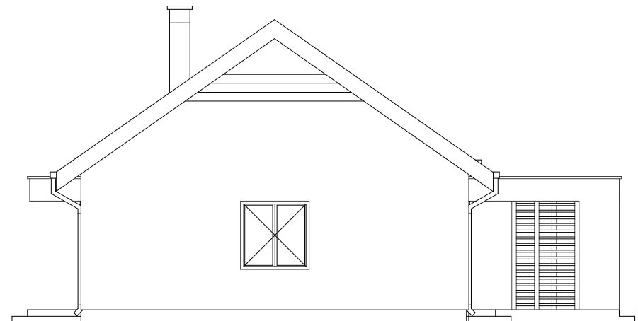
ELEWACJA BOK 2
