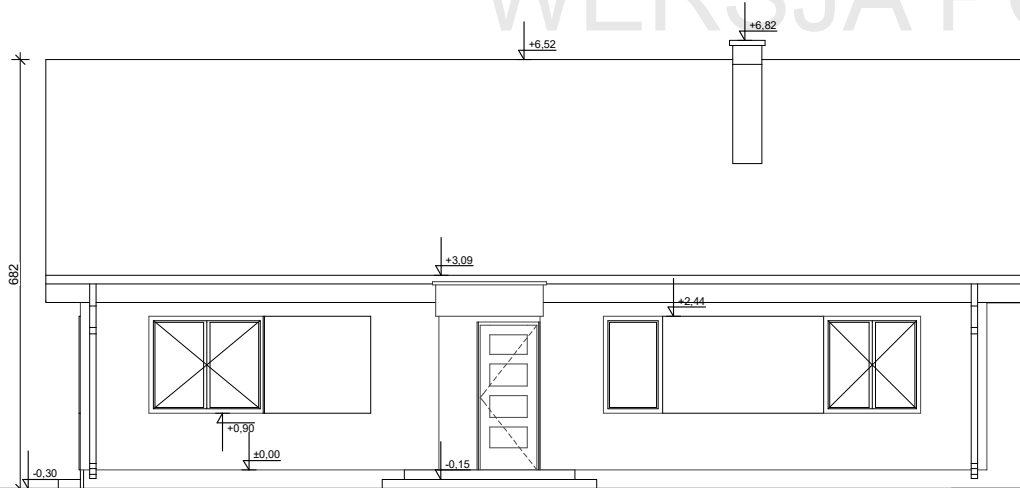
ELEWACJA FRONTOWA
