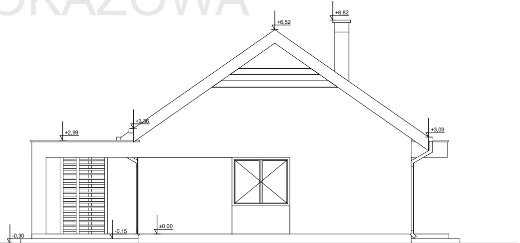
ELEWACJA BOK 1
