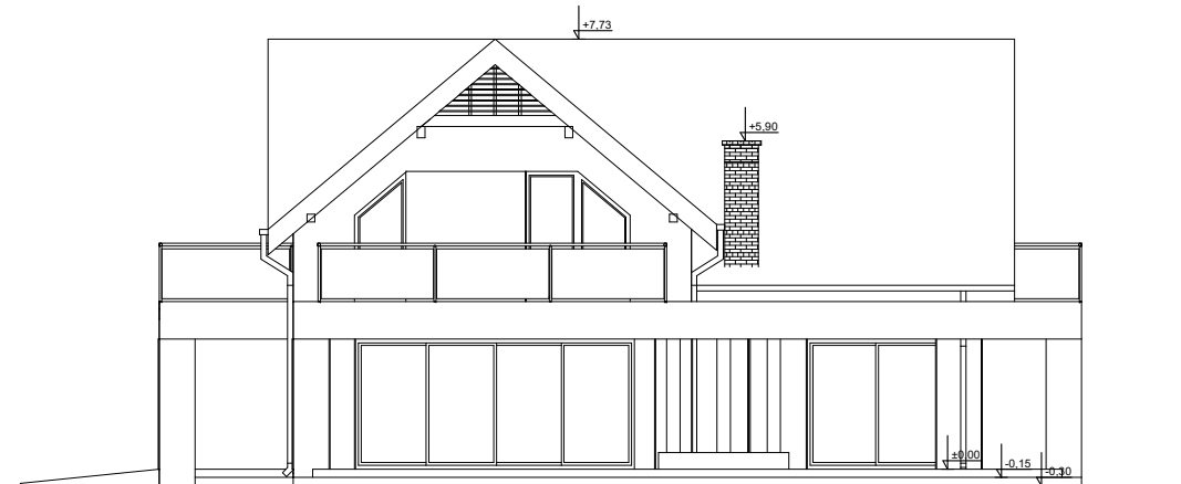
ELEWACJA BOK 2
