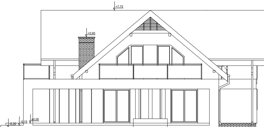
ELEWACJA OGRODOWA
