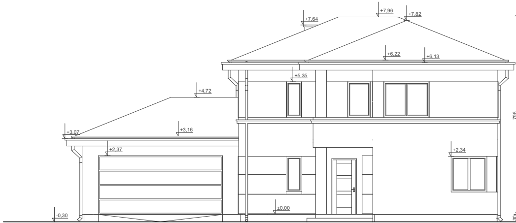
ELEWACJA FRONTOWA
