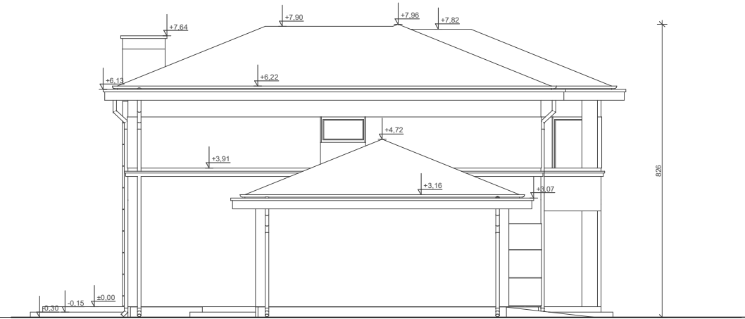
ELEWACJA BOK 1
