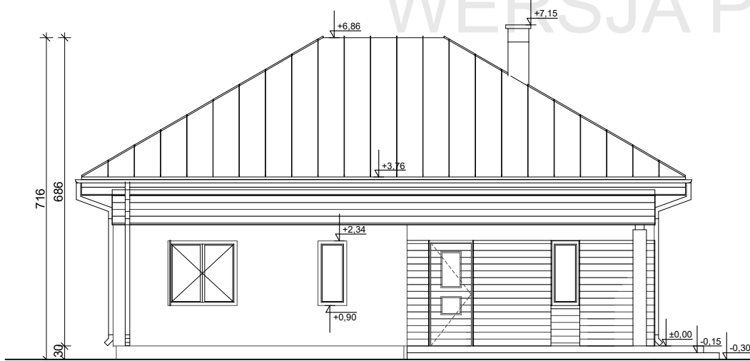
ELEWACJA FRONTOWA
