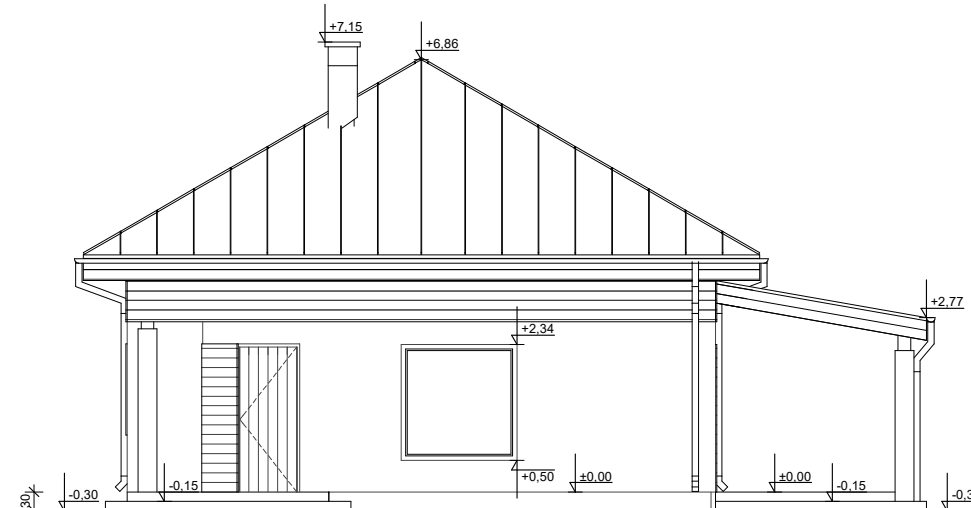
ELEWACJA BOK 2
