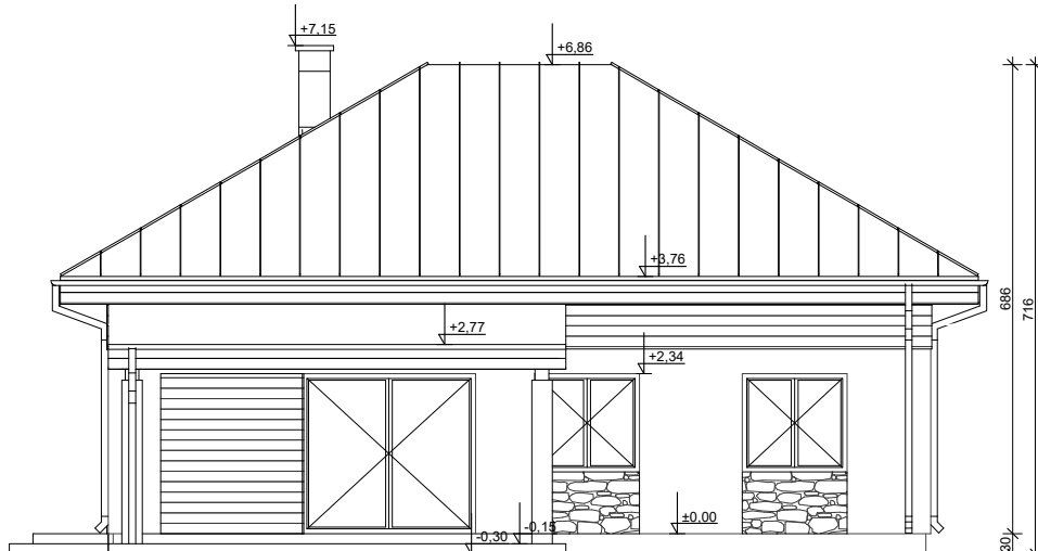
ELEWACJA OGRODOWA
