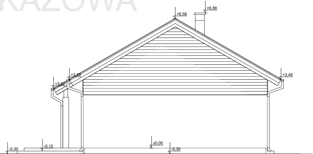
ELEWACJA BOK 1
