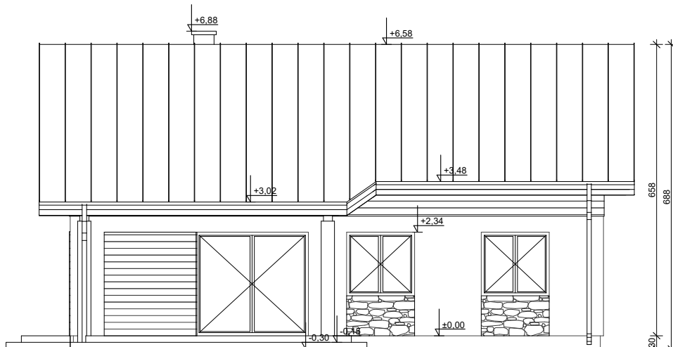
ELEWACJA OGRODOWA
