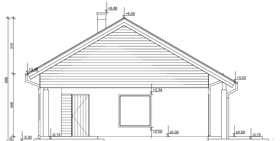
ELEWACJA BOK 2
