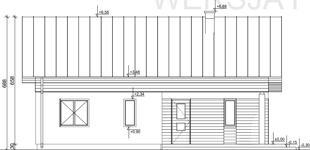
ELEWACJA FRONTOWA
