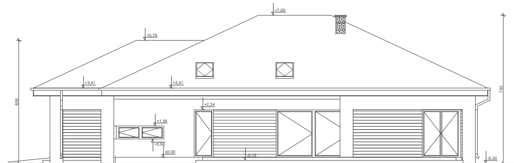
ELEWACJA BOK 2
