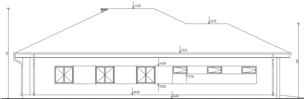
ELEWACJA BOK 1
