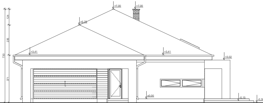
ELEWACJA FRONTOWA
