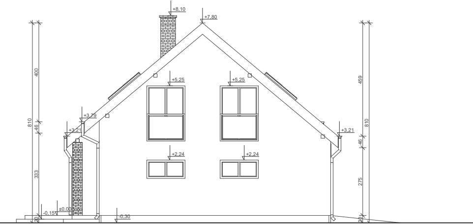
ELEWACJA BOK 1
