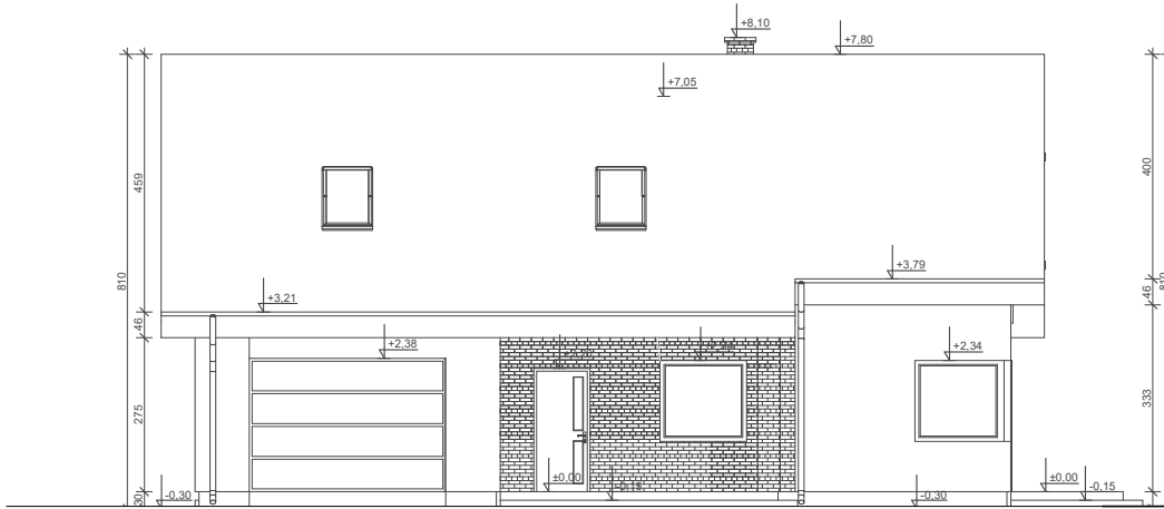
ELEWACJA FRONTOWA
