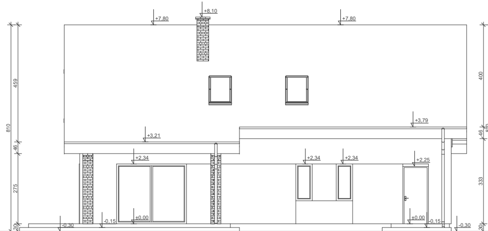
ELEWACJA OGRODOWA
