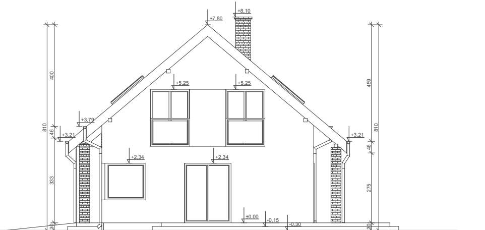
ELEWACJA BOK 2
