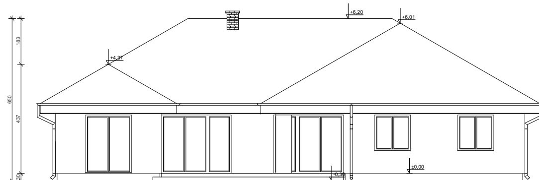
ELEWACJA OGRODOWA
