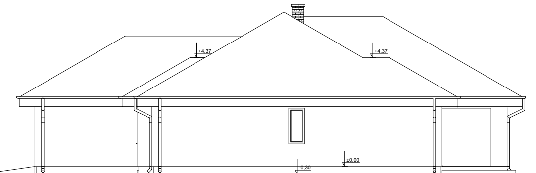
ELEWACJA BOK 2
