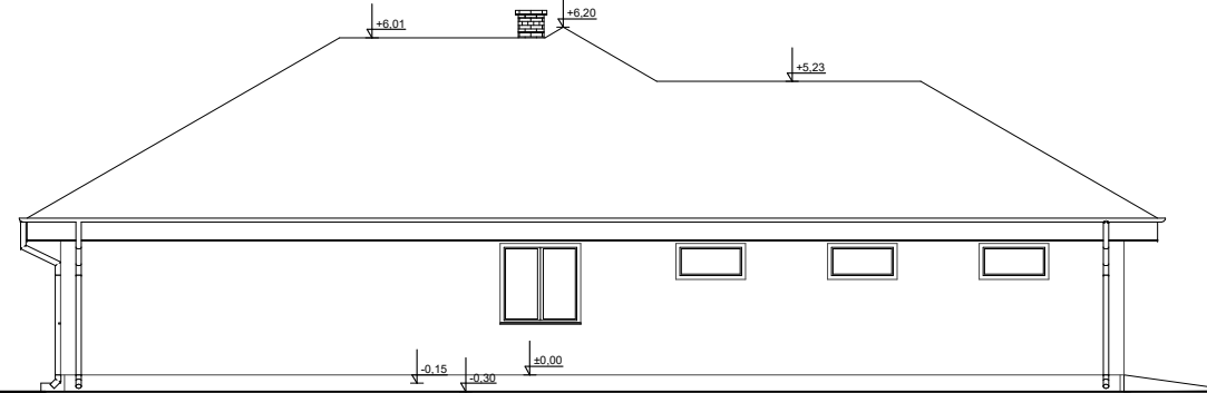
ELEWACJA BOK 1
