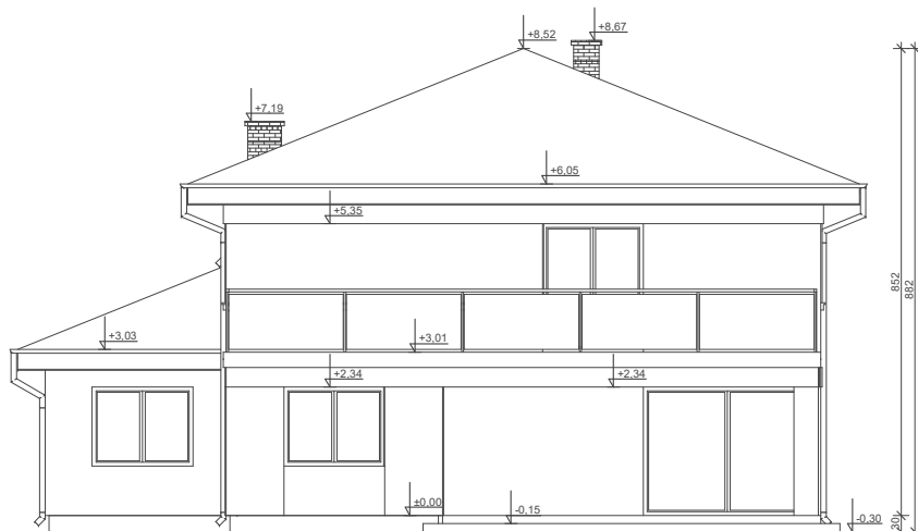
ELEWACJA OGRODOWA
