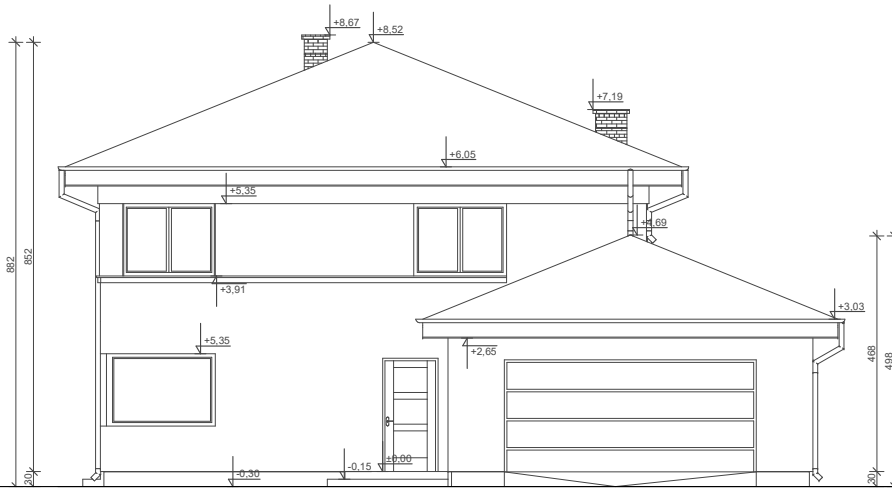
ELEWACJA FRONTOWA
