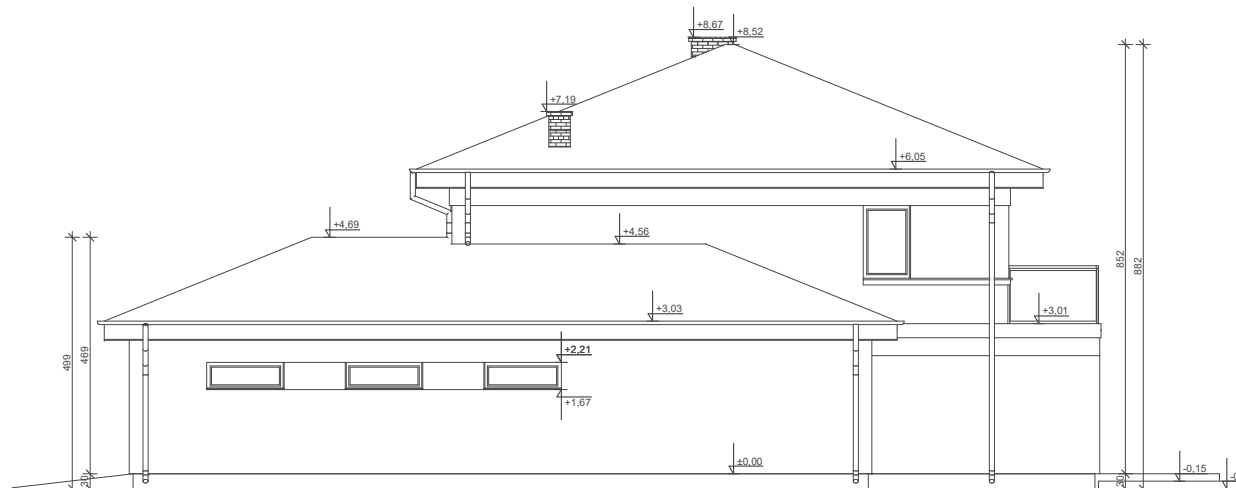
ELEWACJA BOK 2
