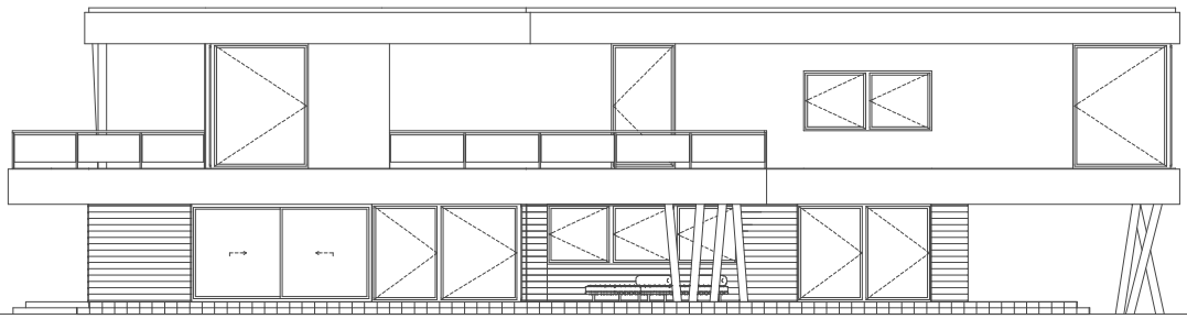
ELEWACJA OGRODOWA
