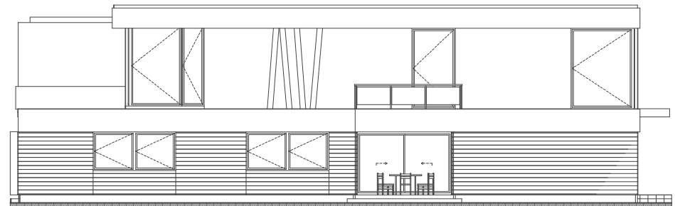
ELEWACJA BOK 2
