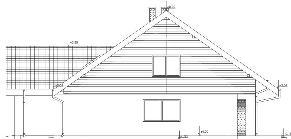
ELEWACJA BOK 2
