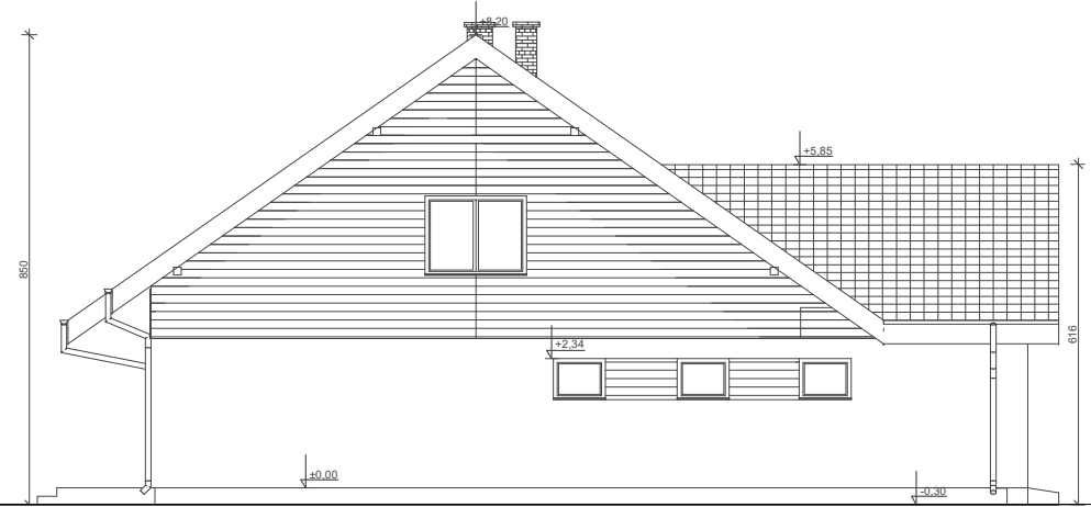
ELEWACJA BOK 1
