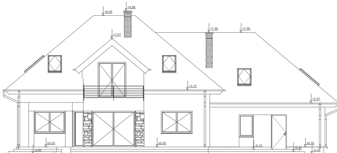
ELEWACJA OGRODOWA
