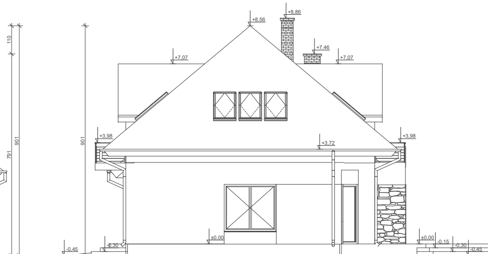
ELEWACJA BOK 2
