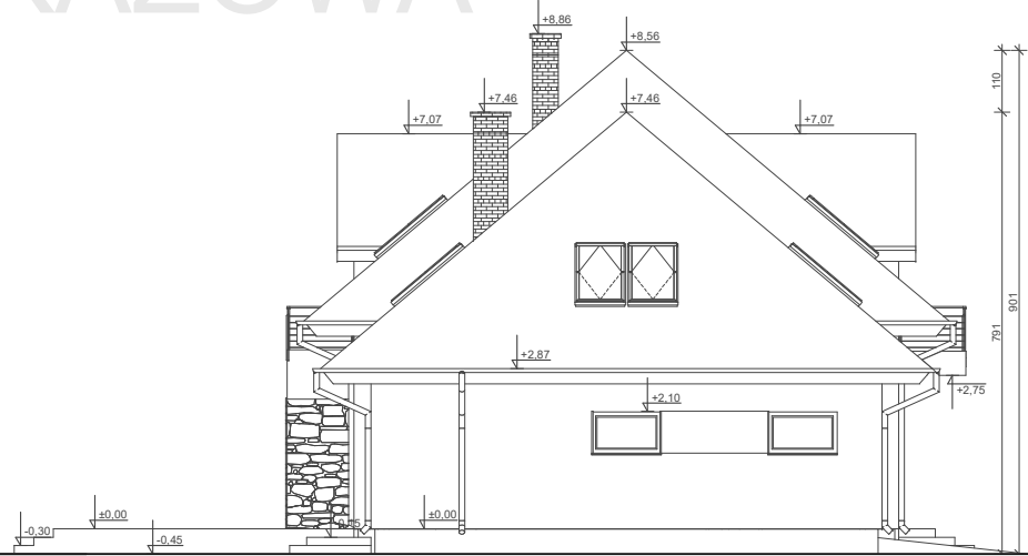
ELEWACJA BOK 1
