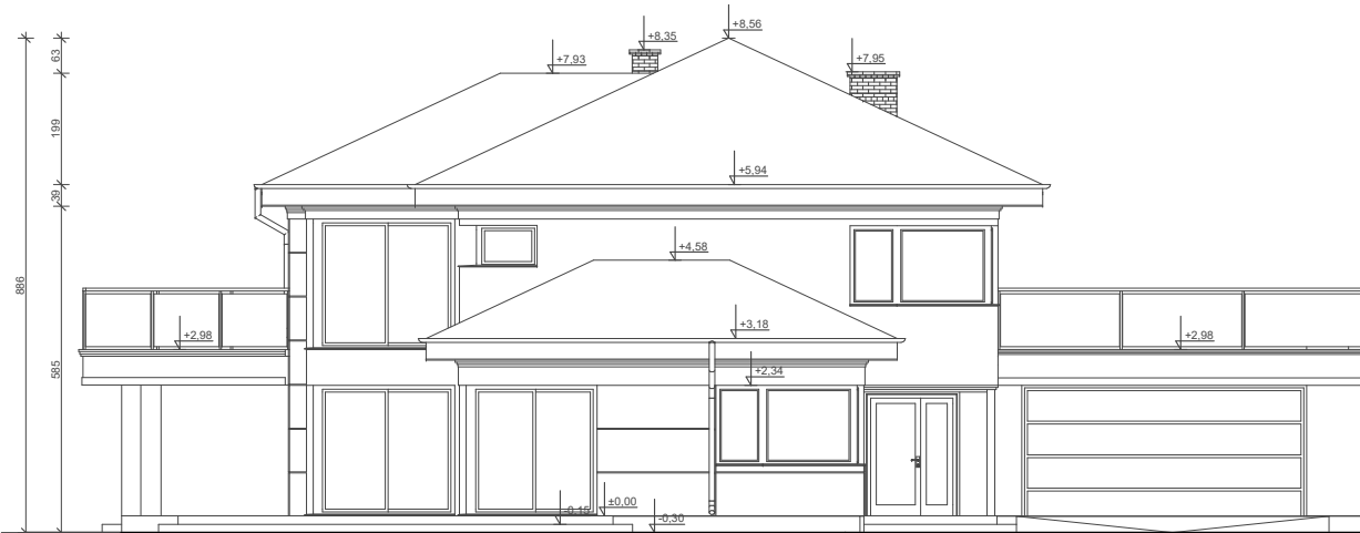
ELEWACJA FRONTOWA
