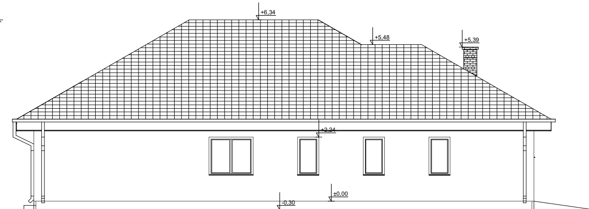
ELEWACJA BOK 2
