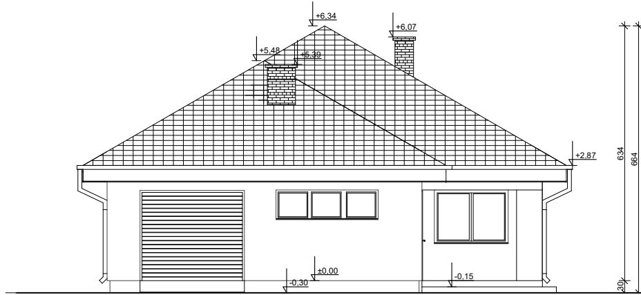
ELEWACJA FRONTOWA
