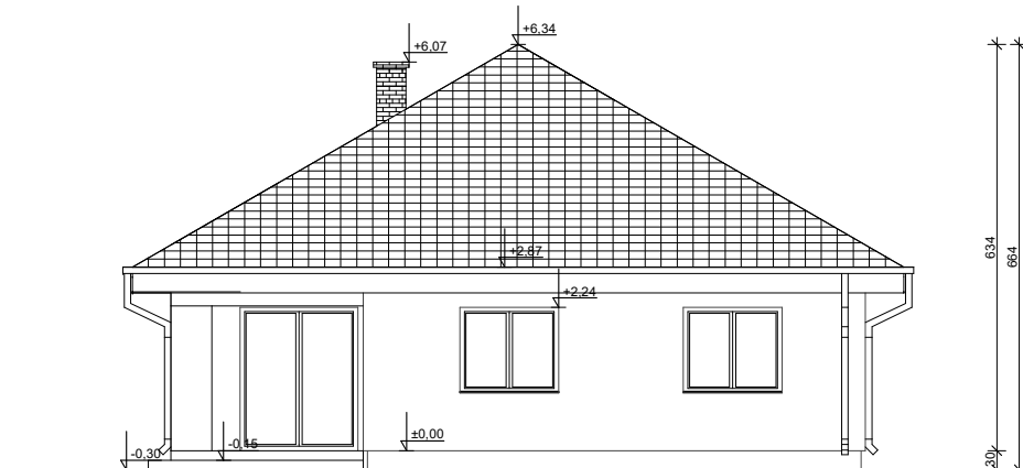
ELEWACJA OGRODOWA
