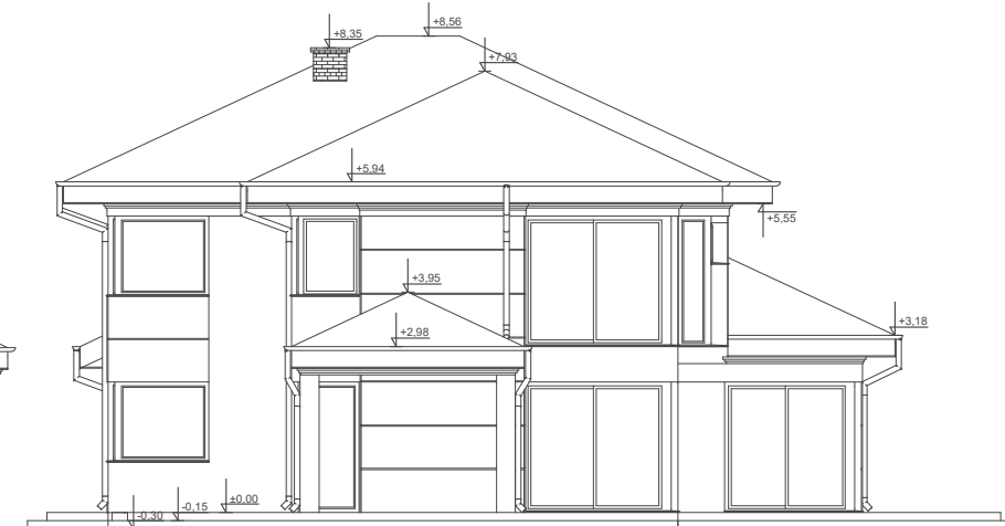
ELEWACJA BOK 2
