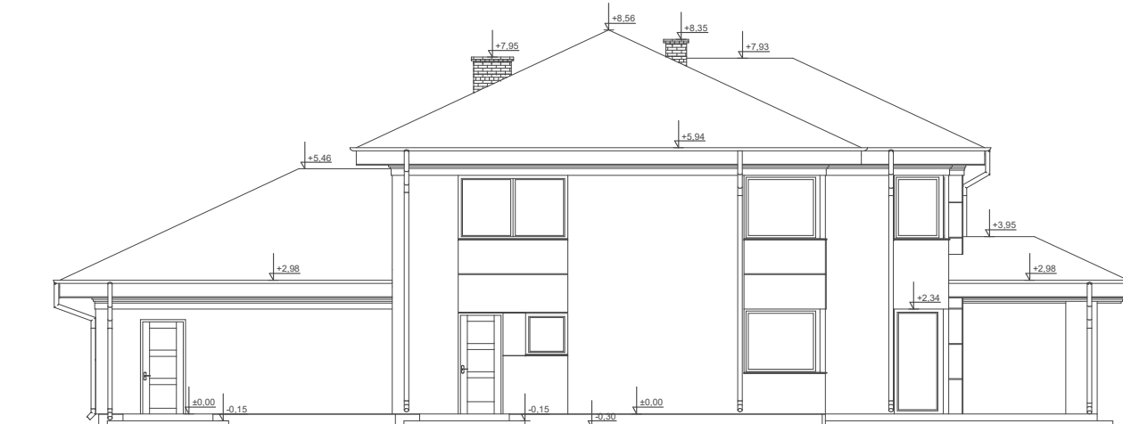
ELEWACJA OGRODOWA
