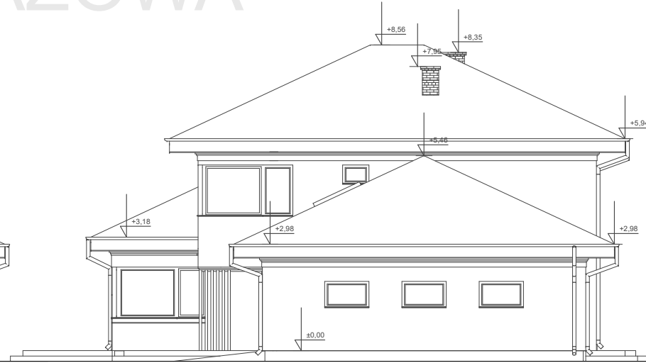
ELEWACJA BOK 1
