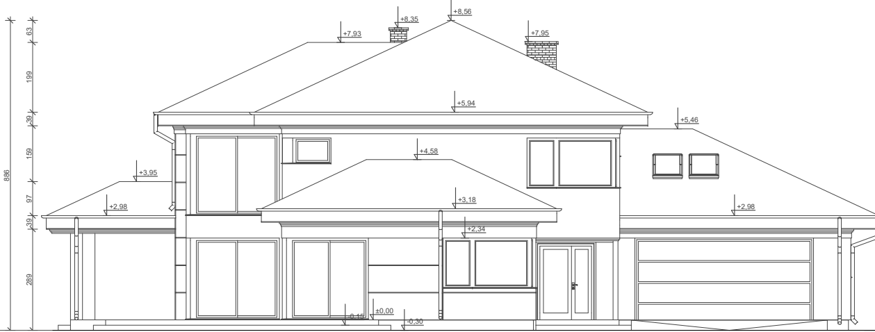
ELEWACJA FRONTOWA
