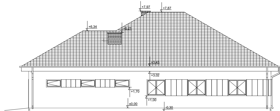
ELEWACJA BOK 2
