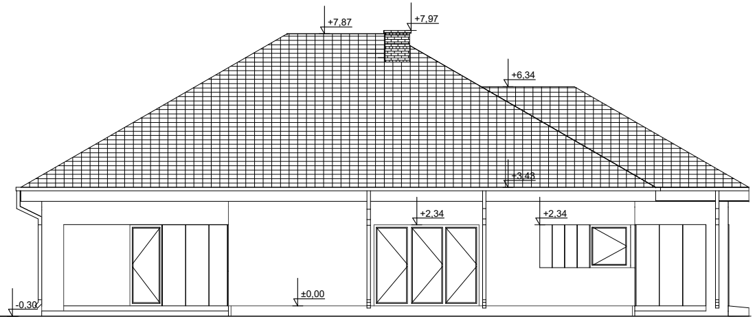
ELEWACJA BOK 1
