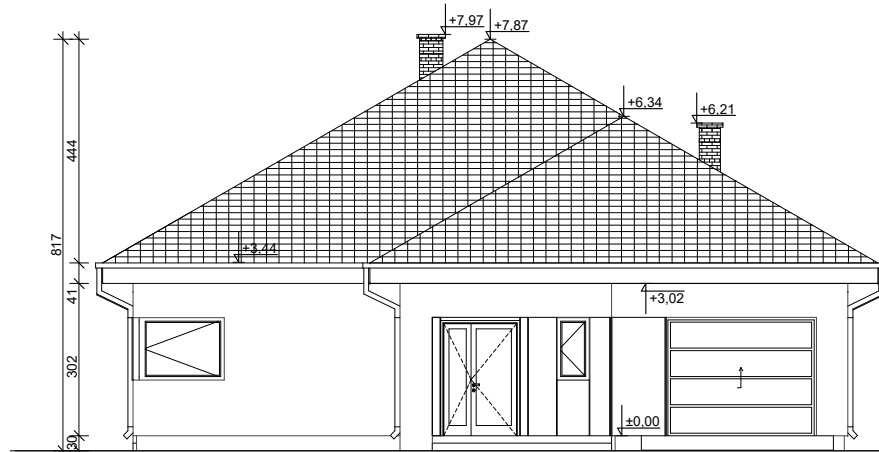
ELEWACJA FRONTOWA
