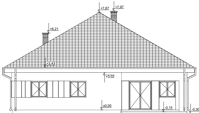
ELEWACJA OGRODOWA
