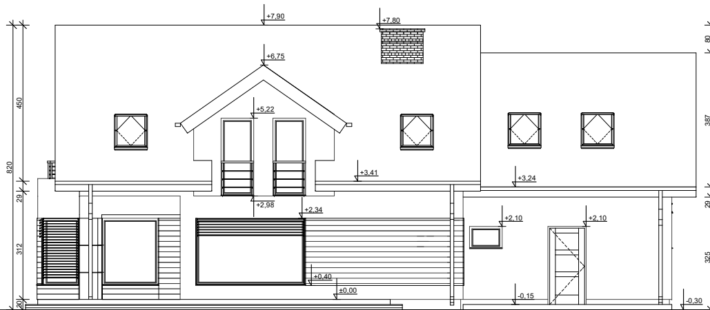
ELEWACJA OGRODOWA
