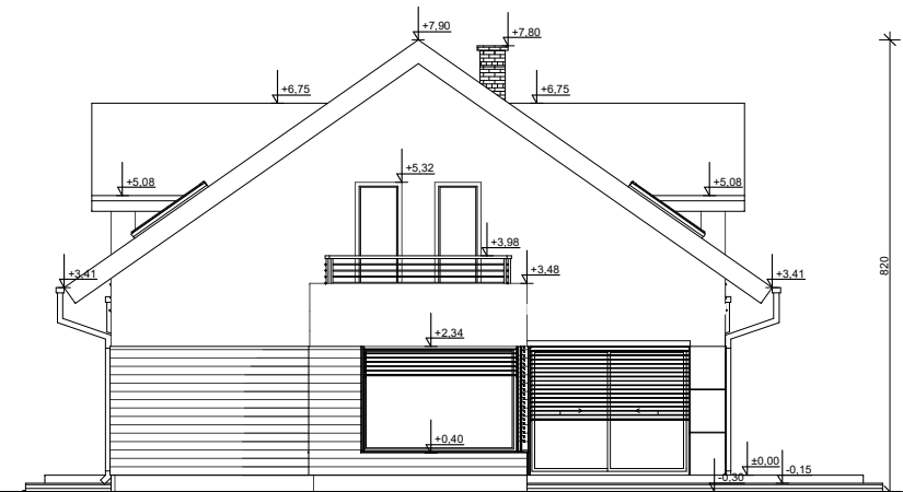
ELEWACJA BOK 2
