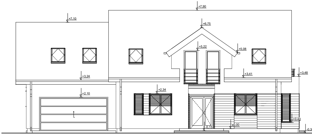
ELEWACJA FRONTOWA
