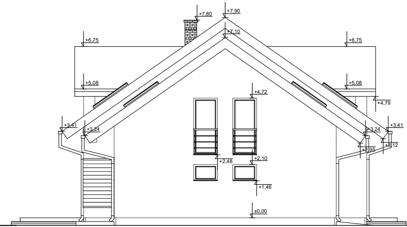
ELEWACJA BOK 1
