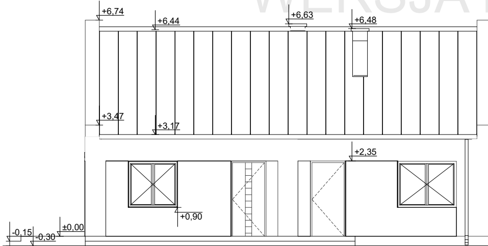
ELEWACJA FRONTOWA
