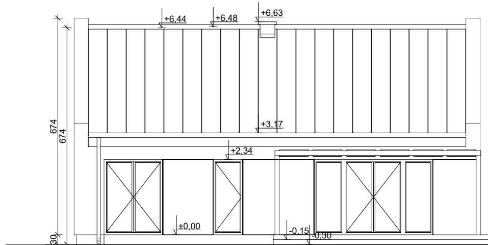
ELEWACJA OGRODOWA
