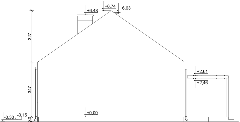
ELEWACJA BOK 2
