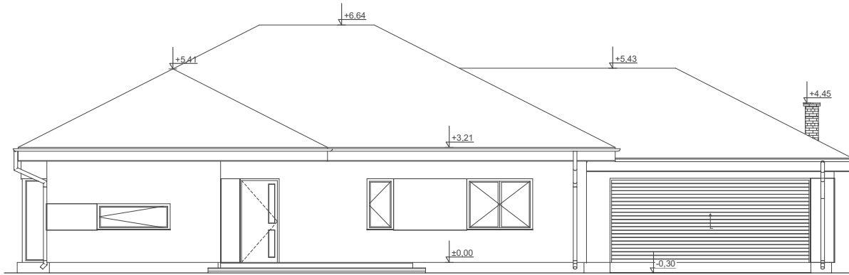
ELEWACJA FRONTOWA
