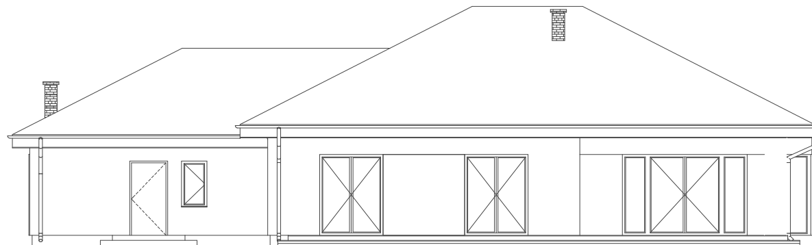
ELEWACJA OGRODOWA
