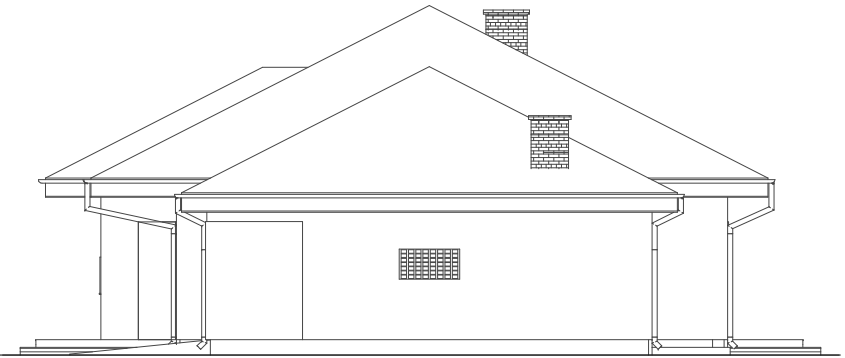
ELEWACJA BOK 1
