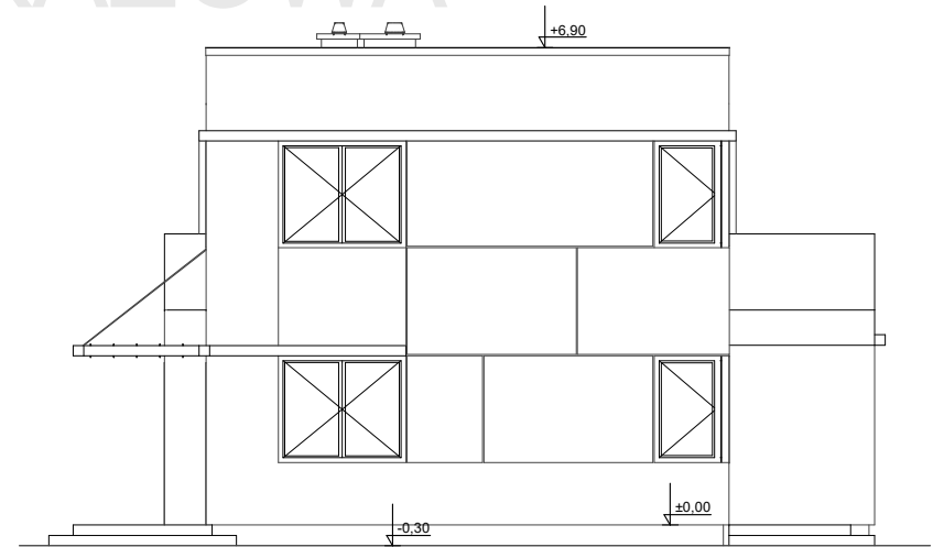
ELEWACJA BOK 1
