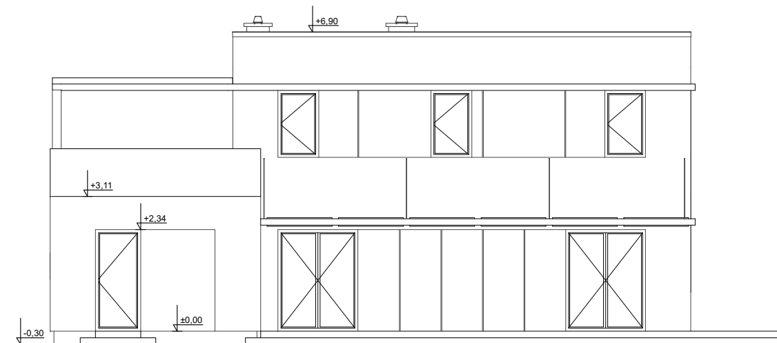
ELEWACJA OGRODOWA
