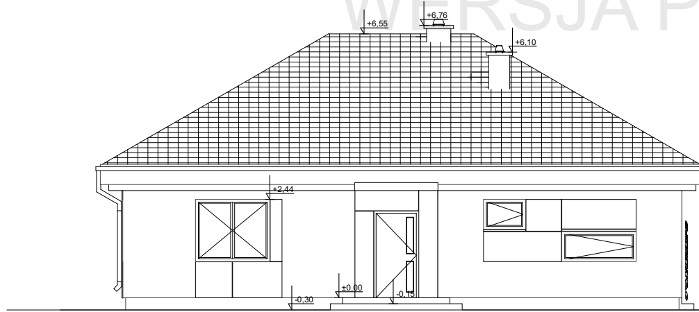
ELEWACJA FRONTOWA
