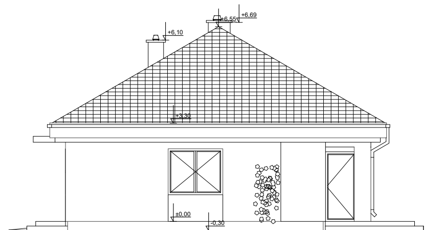
ELEWACJA BOK 2
