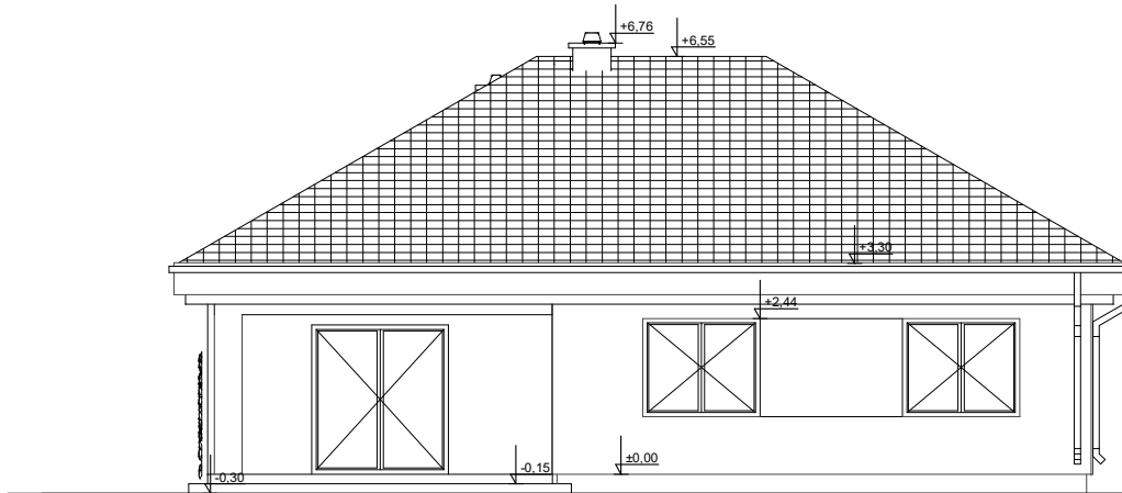
ELEWACJA OGRODOWA
