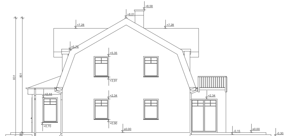
ELEWACJA BOK 2
