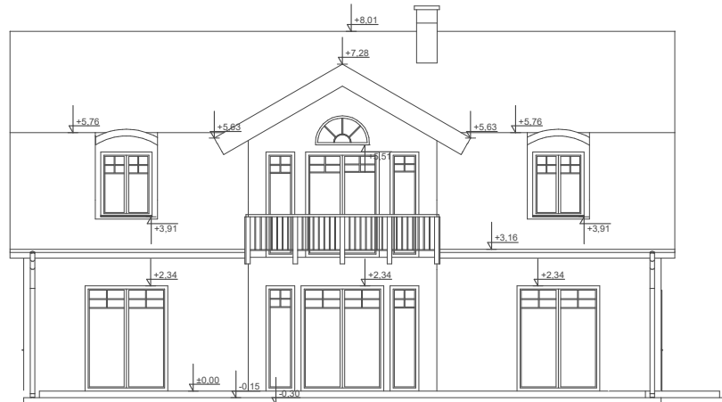
ELEWACJA OGRODOWA
