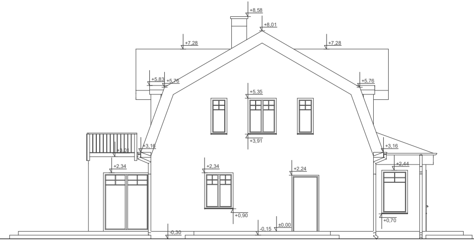
ELEWACJA BOK 1
